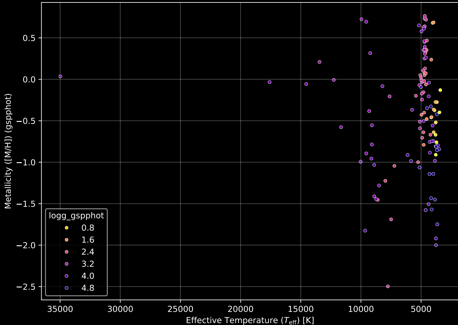
APOGEE DR17 Field: [015+00] Stellar Population Parameters (n= 125)
